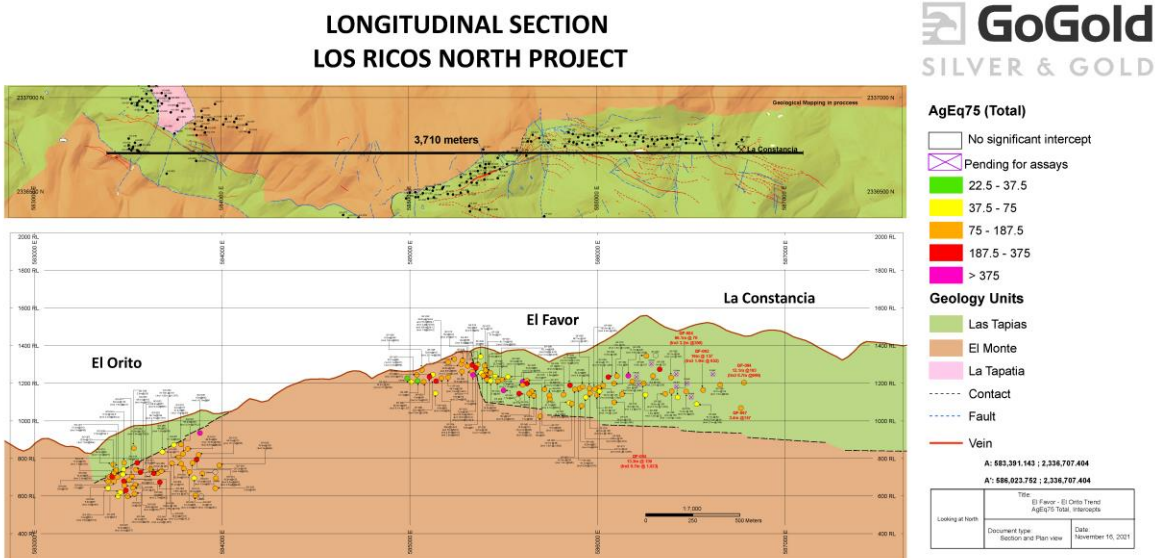
Figure 3: El Favor – El Orito Long Section
